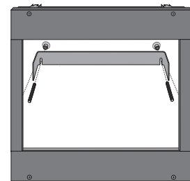
Adapterrahmen 13711 , 200 x 190 mm • zum Einbau von DigitalMonitor 10500X-PLUS in Montageumgebungen mit 190 mm Höhe • incl. Einbaukit 13713 für den Frontplatteneinbau
