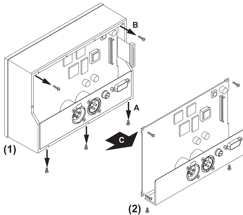
Bild D 7-4: Lösen und Entnehmen von Anschlusswinkel und Hauptplatine
