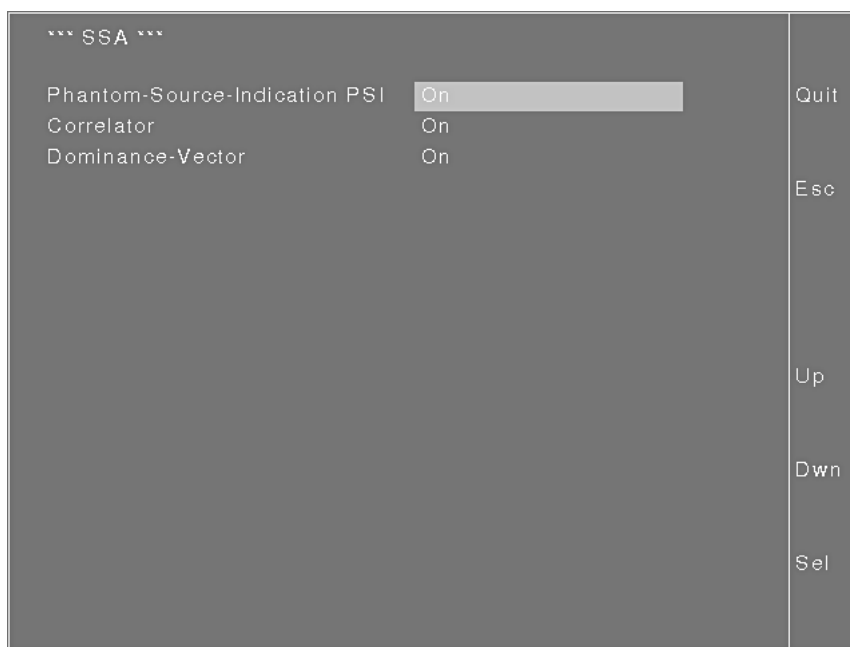
Bild D 4-11: Menü „Sterep“ mit den Stereo-Sound-Analyzer-Parametern
