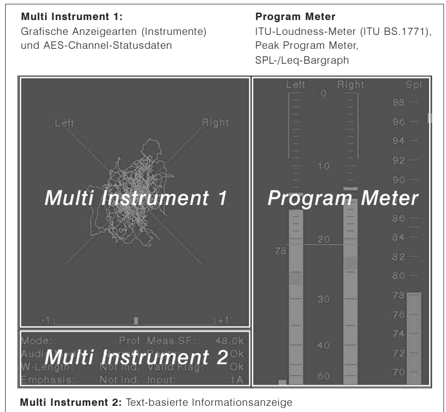
Bild D 2-1: Die Displayelemente des DigitalMonitor 10500X-PLUS
