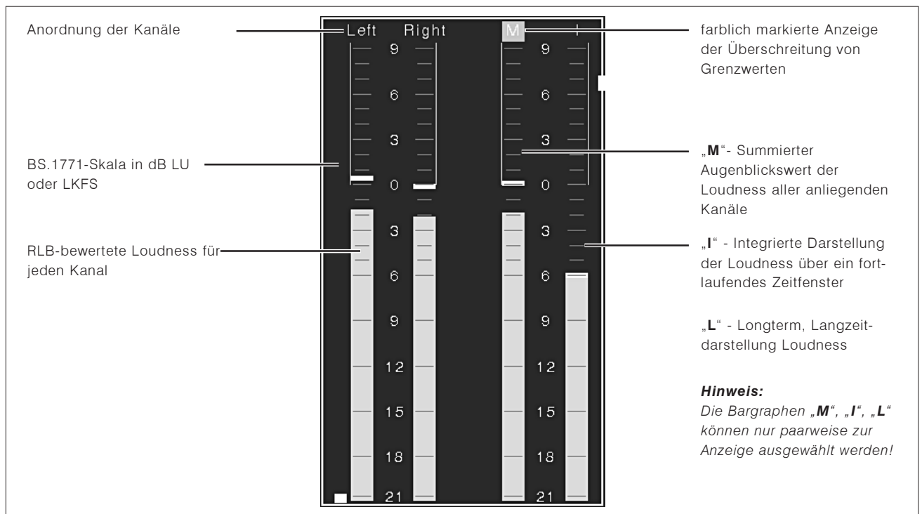
Bild D 4-4: Die „Program Meter“-Anzeige im ITU BS.1771-Modus (Loudness)
