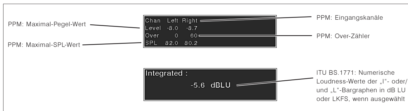
Bild D 4-20: Die numerische Anzeige im „Multi Instrument 2“, oben im „Program Meter“-Modus „PPM“, unten im „Program Meter“-Modus „ITU BS.1771“
