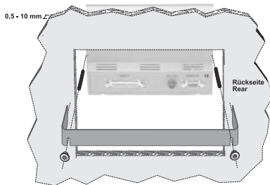
Einbaukit 13713 für den Frontplatteneinbau • Erforderlicher Frontplattenausschnitt: 174,9 x 123,8 mm (B x H) • Plattendicke: 0,5 bis 10 mm (Instrument nicht enthalten)
