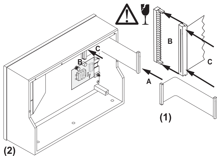
Bild D 7-9: Aufstecken des Flachband-Anschlusskabels auf die Displayplatine
