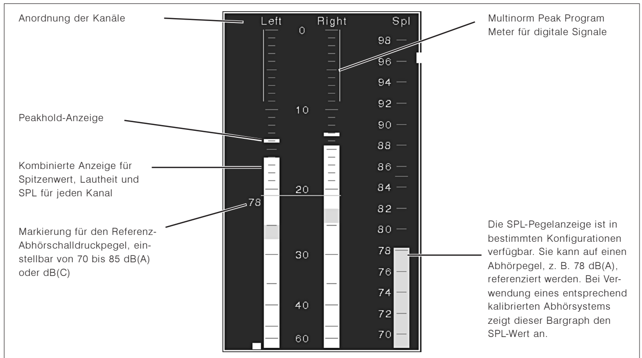
Bild D 4-1: Die „Program Meter“-Anzeige im PPM-Modus
