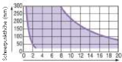
Kameraplattform Counterbalance
